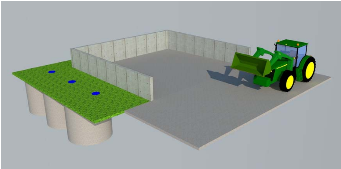
Joonis 15. II tüüpi tahesõnnikuhoidla eskiis
