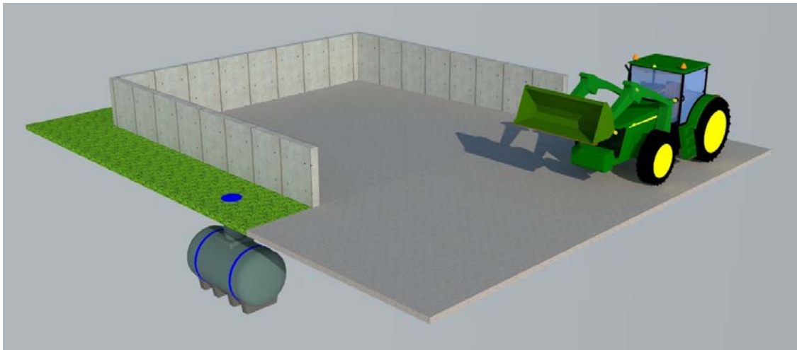
Joonis 13. I tüüpi tahesõnnikuhoidla eskiis
