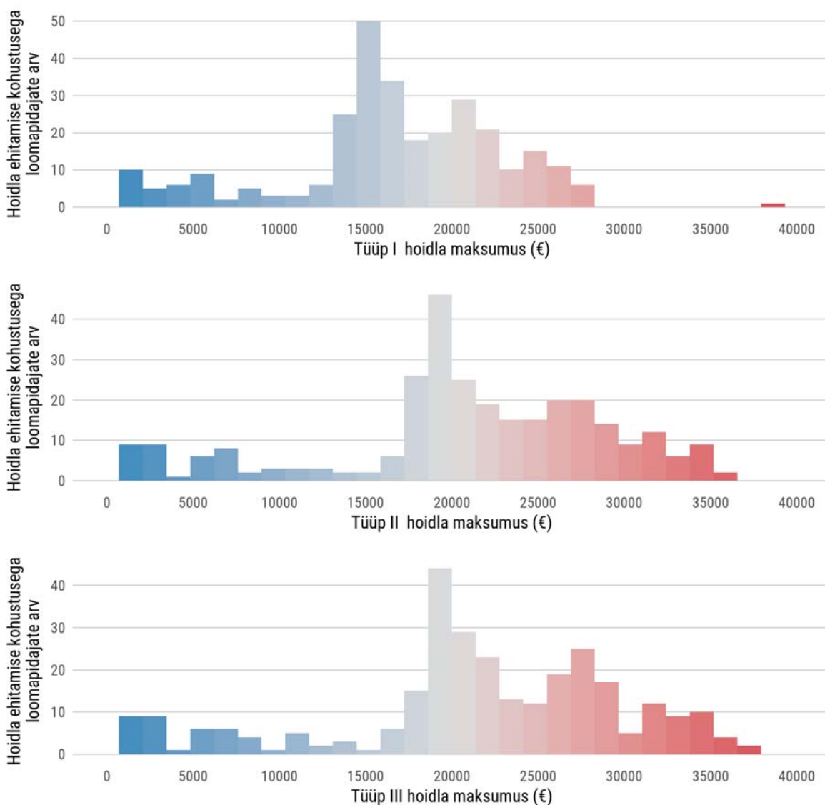
Joonis 17. Mõjutatud loomapidajate jaotus hoidla maksumuse alusel erinevate sõnnikuhoidla tüüpide võrdluses
